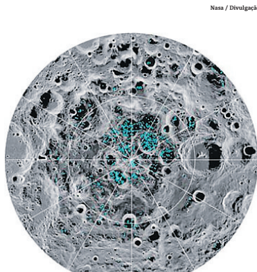
Superfícies de gelo estão nas áreas mais escuras da Lua
