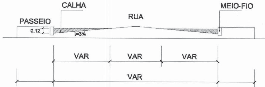
Perfil Transversal Típico de via
