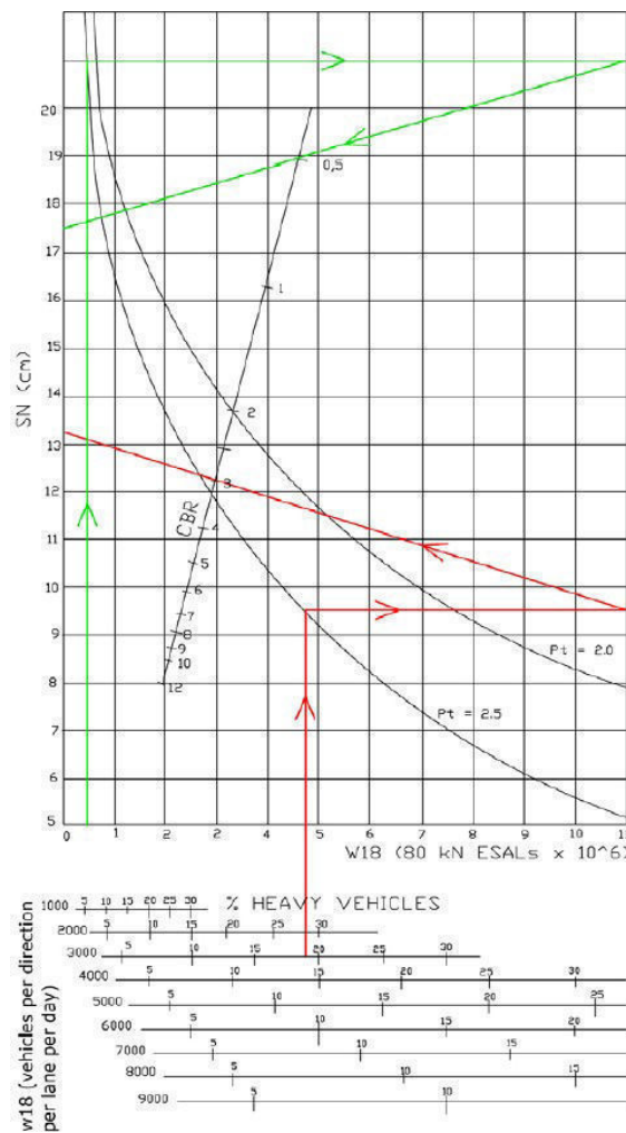
Figura 14: TráfegototalW18versusNúmeroEstruturalSN.
