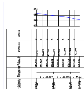
RUA PROJETADA J
