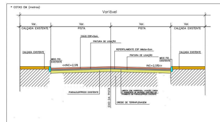
SEÇÃO TRANSVERSAL TÍPICA-RUA PROJETADA I
