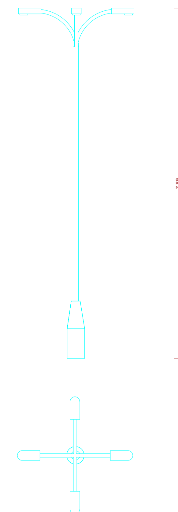
POSTE CONCRETO SEÇÃO CIRCULAR COMPRIMENTO=9M 4 PÉTALAS
