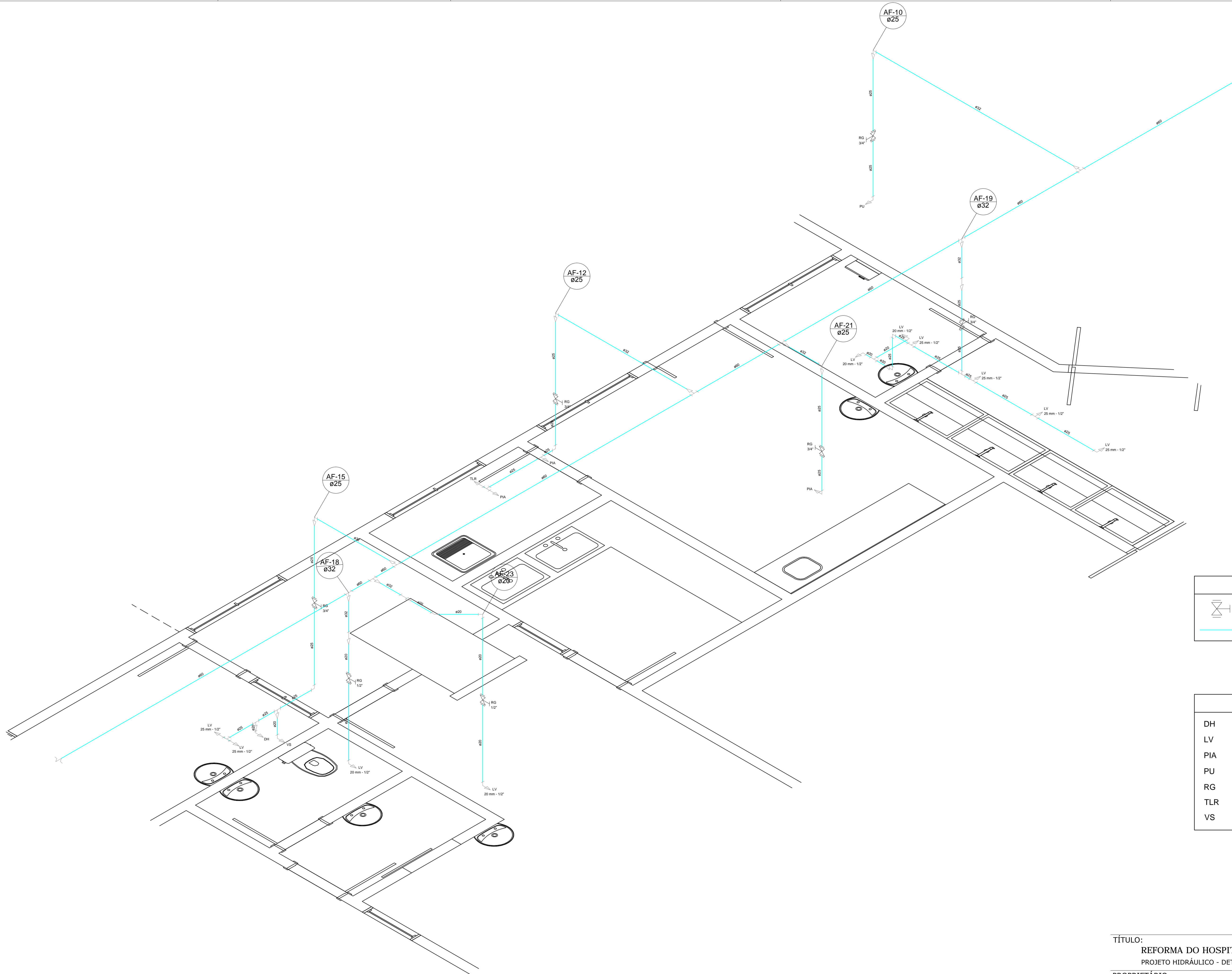
Detalhe Isométrico - H4 Escala 1:25
